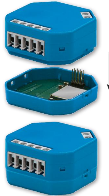
Baureihe 64 mit EnOcean-Adapter EOA64
